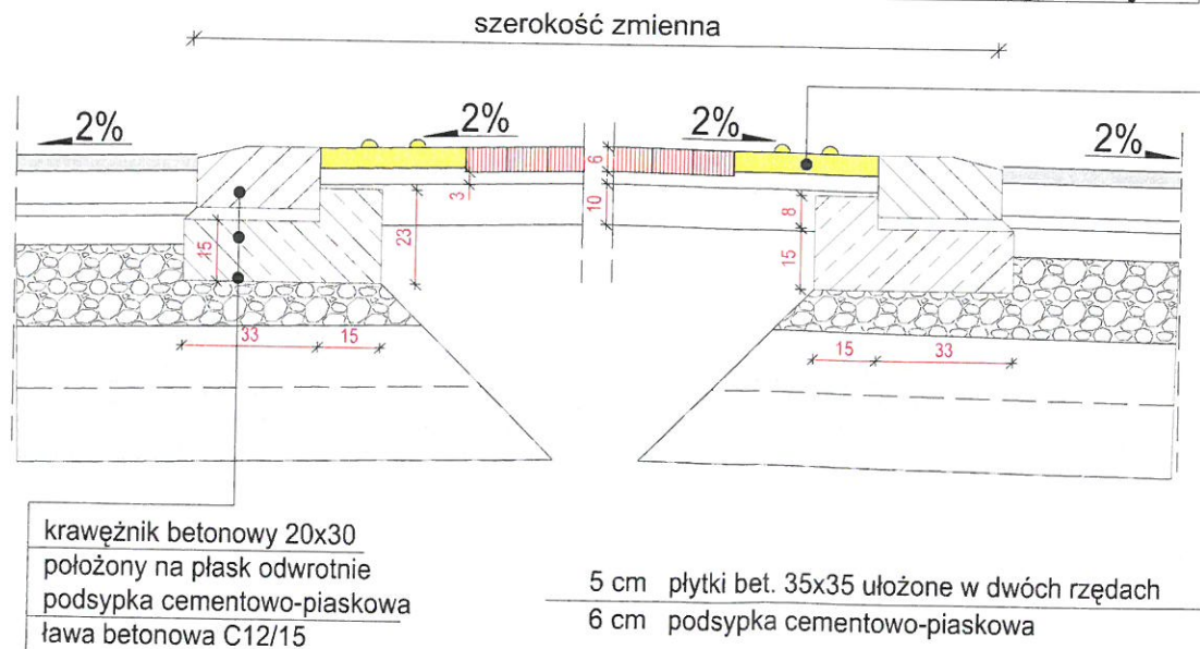
Szczegół wykonania wyspy dzielącej z przejściem dla pieszych
