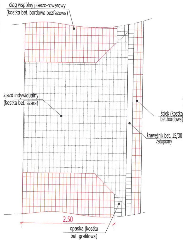
Plan nawierzchni w obrębie zjazdu typ A
