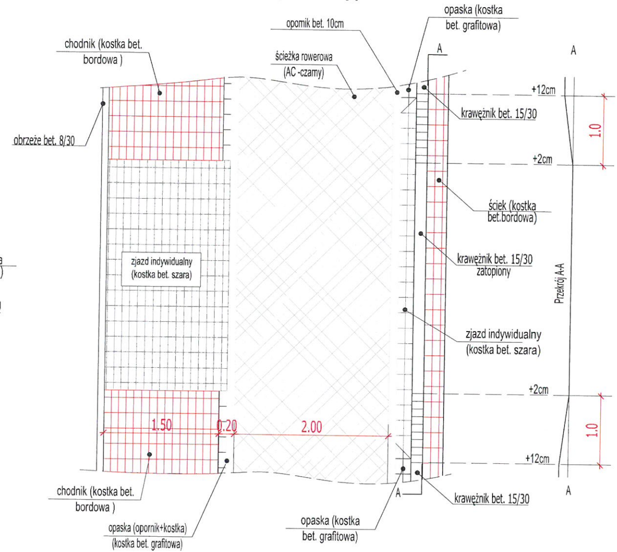
Plan nawierzchni w obrębie zjazdu typ C
