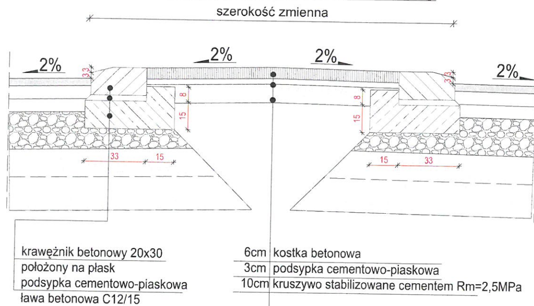
Szczegół wykonania wyspy dzielącej
